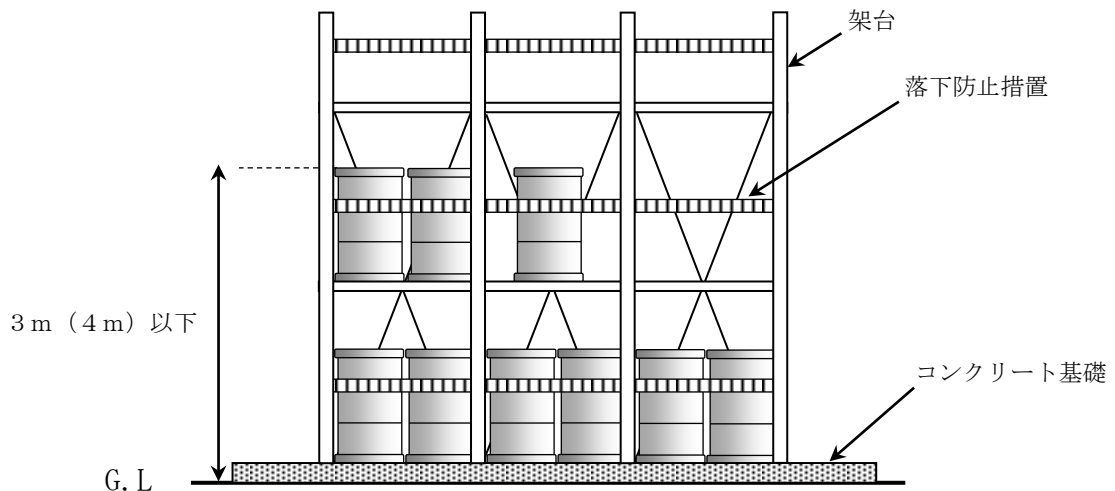
第4-6-2図 架台の構造
