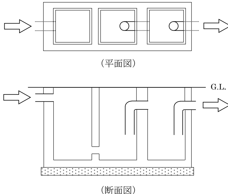
第 4-5-3 図 ためますを含めた油分離槽
